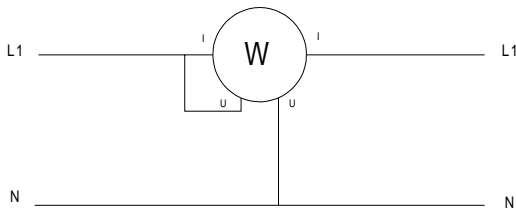
Fig 4.4.1 Schema di collegamento in monofase
