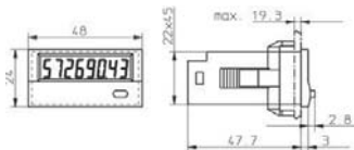
Dimensioni CODIX 140 e 142
