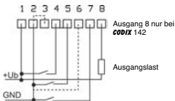
Belegung der Anschlussklemmen
