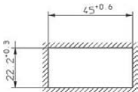
Schalttafelauausschnitt CODIX 140 und 142
