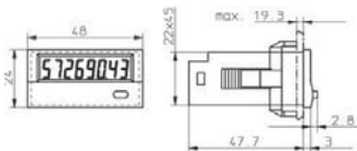
Maßbild CODIX 140 und 142
