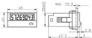
Dimensiones CODIX 140 y 142
