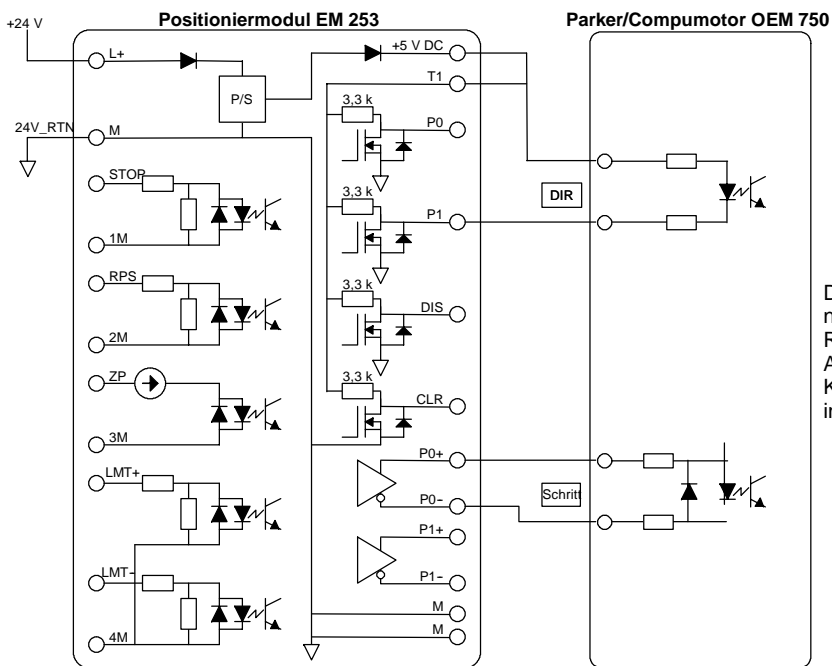
Bild A-36 Anschließen eines Positioniermoduls EM 253 an ein Parker/Compumotor OEM 750
