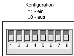
Bild A-21 DIP-Schalter des EM 231 RTD-Modul
