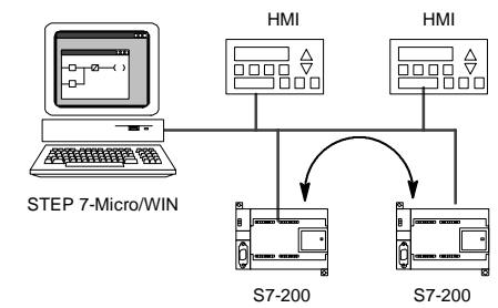
Bild 7-13 Punkt-zu-Punkt-Kommunikation
