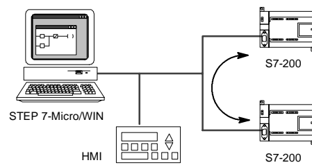
Bild 7-13 Punkt-zu-Punkt-Kommunikation
