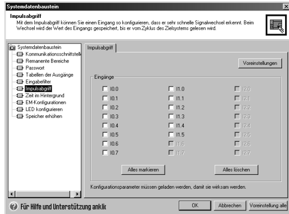
Bild 4-24 Impulsabgriff
