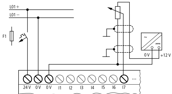
Abbildung 19: Sollwertgeber
