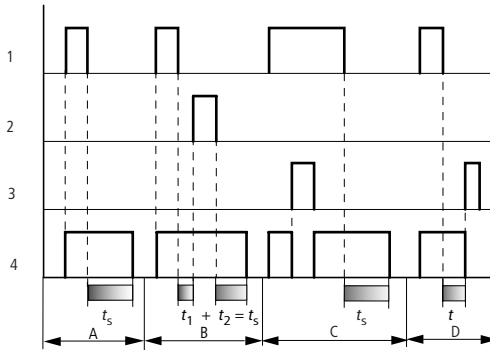
Abbildung 107: Wirkdiagramm Zeitrelais rückfallverzögert (mit/ohne Zufallsschalten, mit/ohne Retriggerung)
