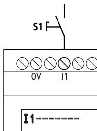
Abbildung 125:easy-Eingang mit Schalter belegt
