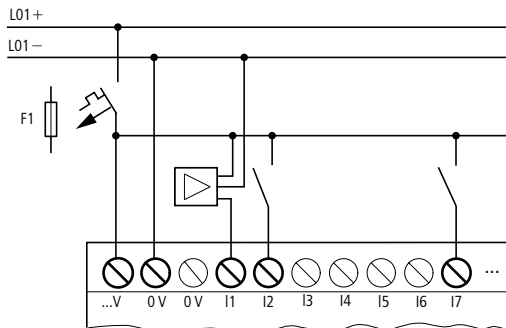
Abbildung 17: easy-DC
