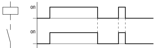
Abbildung 60: Wirkdiagramm Schützfunktion
