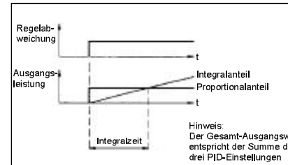
Bild 8.2: Integralzeit
