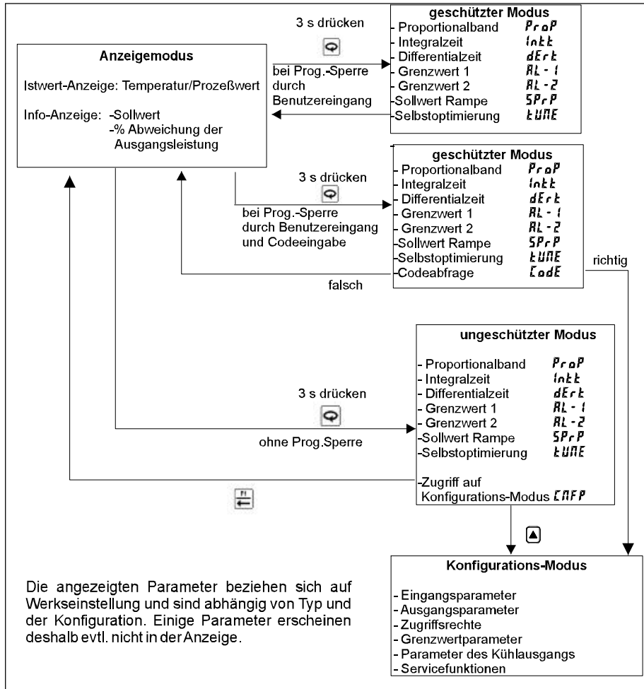
Bild 6.1: Eingabeebenen
