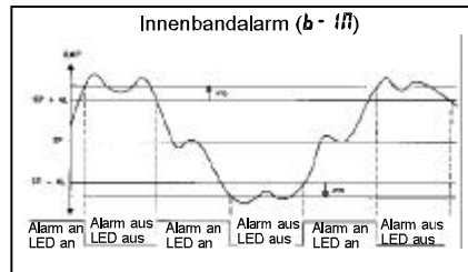
Bild 7.6: Innenbandalarm
