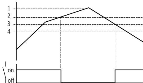
Abbildung 49: Wirkdiagramm Analogwertvergleicher Betriebsart „kleiner als“
