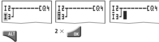
Abbildung 39: Kontakt I1 von Schließer zu Öffner ändern
