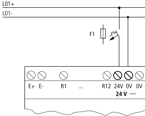
Abbildung 10: Versorgungsspannung an DC-Erweiterungsgeräte
