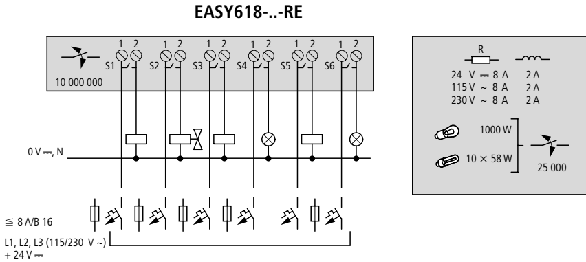
Abbildung 30: Relais-Ausgänge EASY618-...-RE
