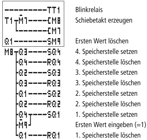
Abbildung 78: easy-Schaltplan Lauflicht
