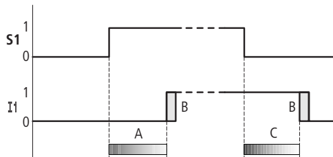
Abbildung 83: Verzögerungszeiten von easy-DC und easy-DA
