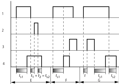
Abbildung 68: Wirkdiagramm Zeitrelais, ansprech- und rückfallverzögert 2
