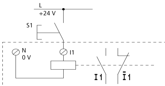
Abbildung 11: Eingänge anschließen
