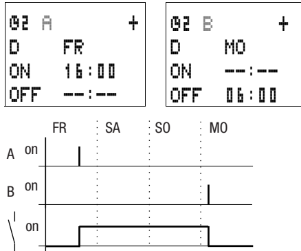
Abbildung 60: Wirkdiagramm „Wochenende“
