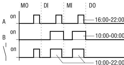
Abbildung 62: Wirkdiagramm „Zeitüberschneidungen“
