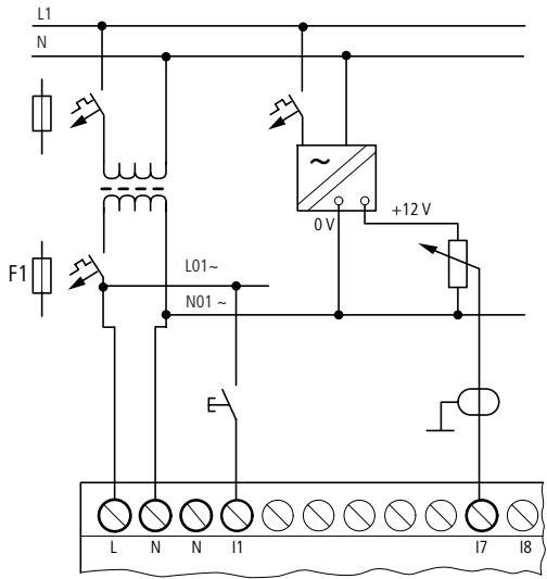
Abbildung 20: easy-AB analoger Eingang, Verbindung der Bezugspotentiale
