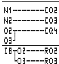
Schaltplandarstellung
