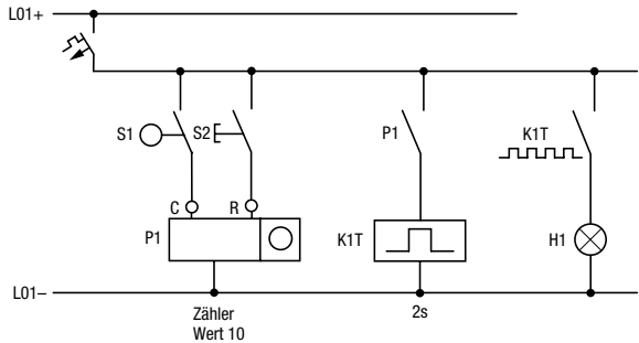
Abbildung 46: Festverdrahtung mit Relais
