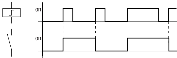
Abbildung 44: Wirkdiagramm Stromstoßrelais
