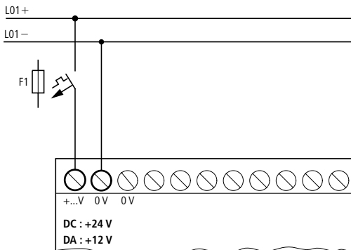
Abbildung 9: Versorgungsspannung an DC-Basisgerät
