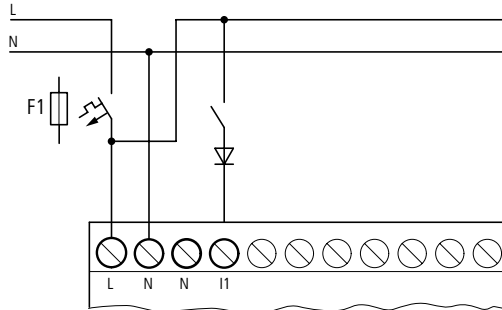
Abbildung 14: AC-Eingang mit Entstörungsdiode easy-AC und easy-AB
