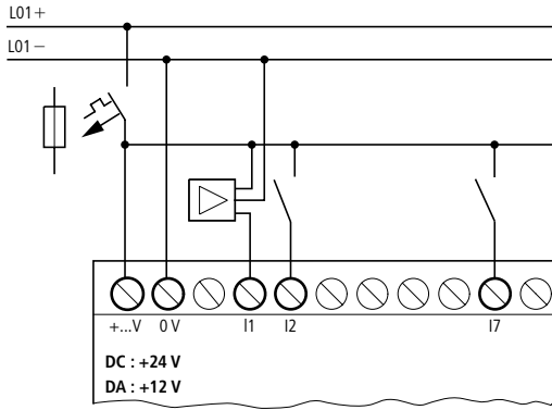
Abbildung 18: Digitale Eingänge anschließen easy-DC, easy-DA
