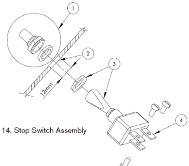
Zusammenbau Abstellschalter
