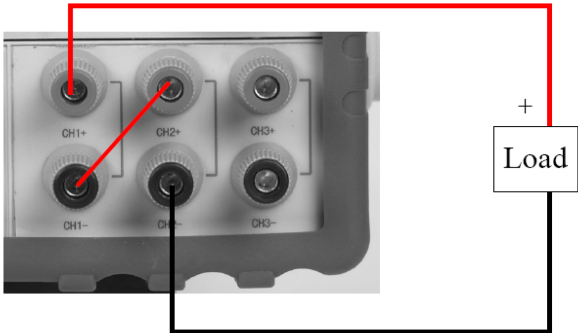
Connexion d'un montage série : exemple voie 1 et 2
