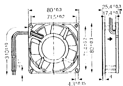
Maßbild
