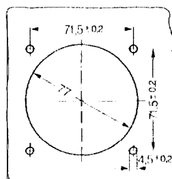
Montagemaße
