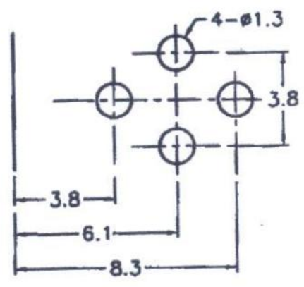
P.C.B LAYOUT
